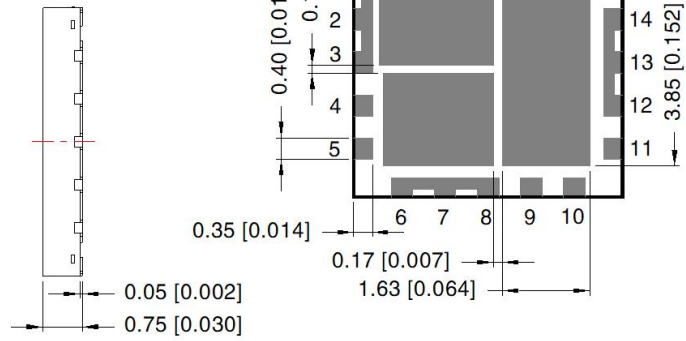
右视图
