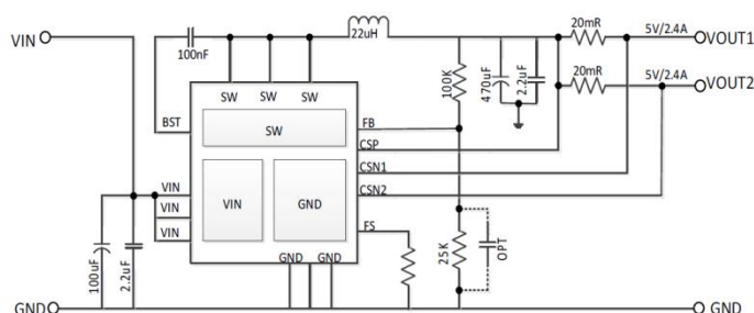
双通道典型应用图
