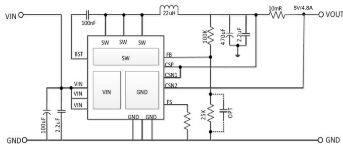
单通道典型应用图
