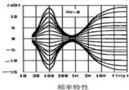
频率特性
